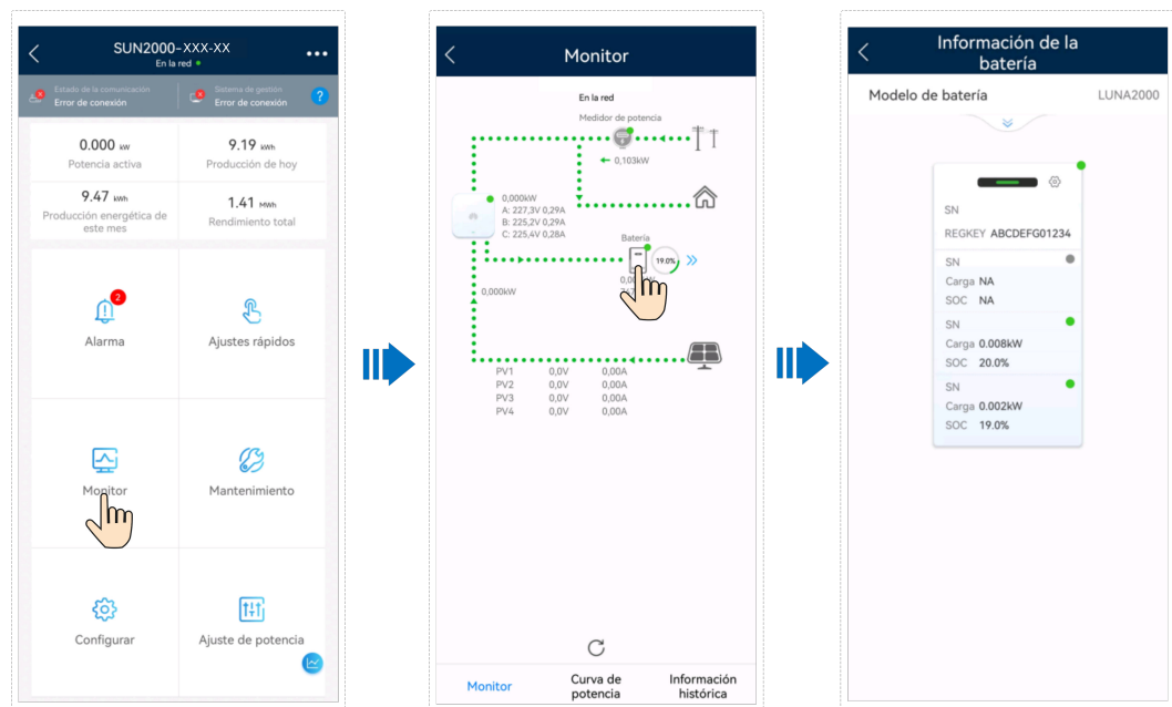
Figura 6-4 Consulta del estado del ESS
