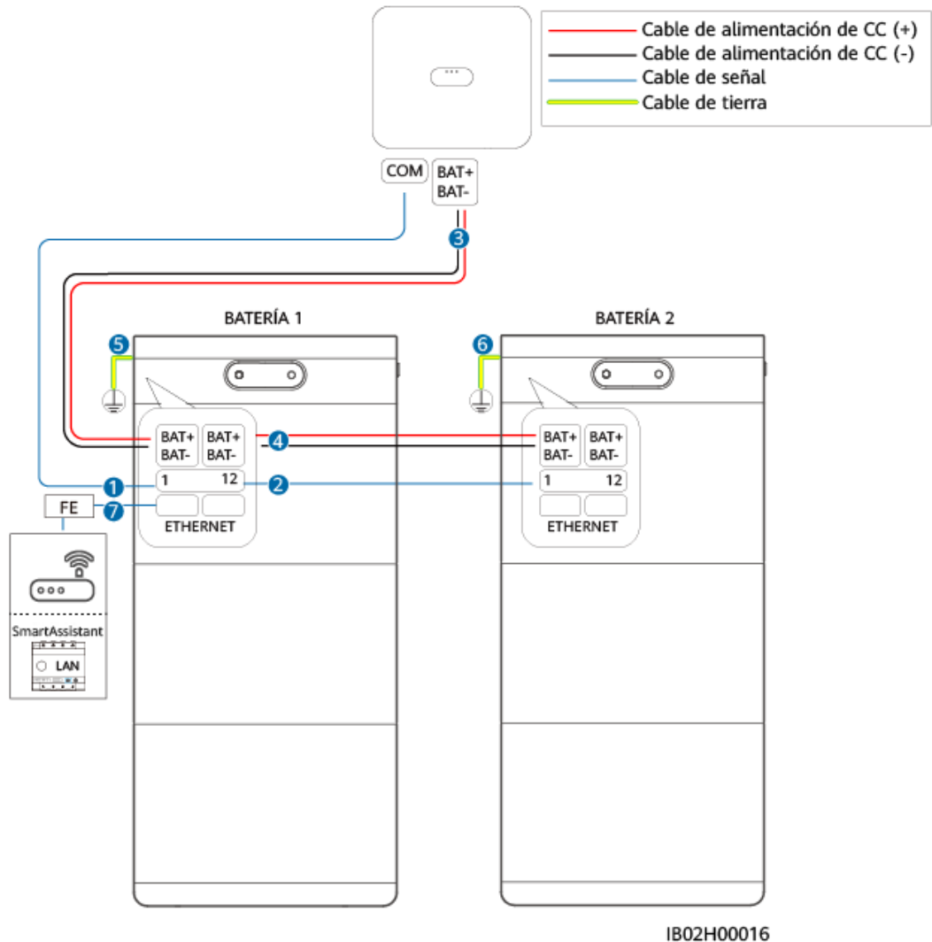
Figura 5-1 Conexiones de los cables del ESS
