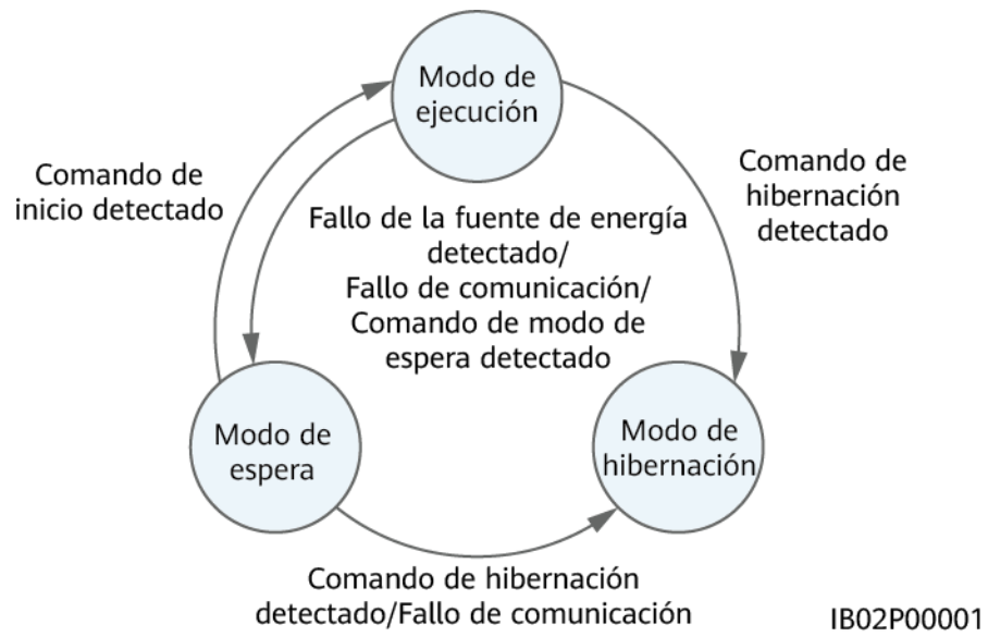
Figura 2-18 Cambio del modo de funcionamiento
