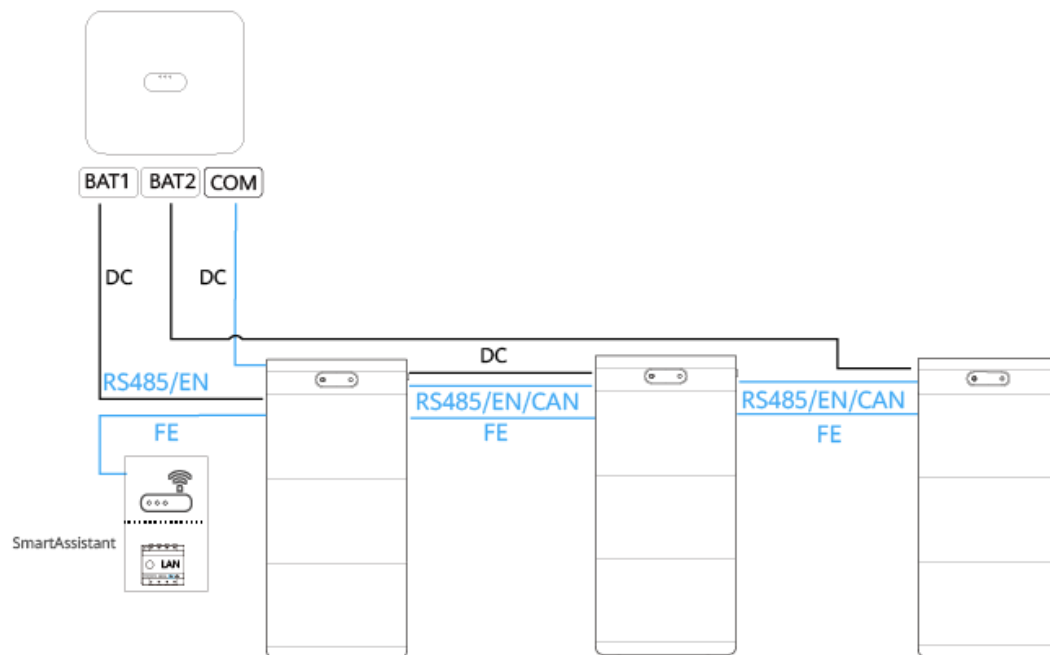
Figura 2-12 Conexión de los ESS al inversor (3)
