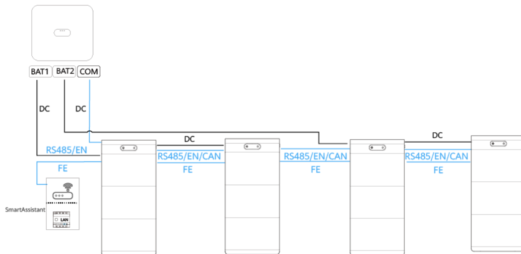
Figura 2-13 Conexión de los ESS al inversor (4)
