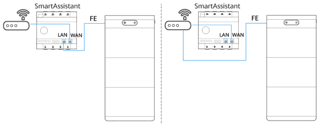
Figura 5-8 Puerto de red conectado al SmartAssistant o al router
