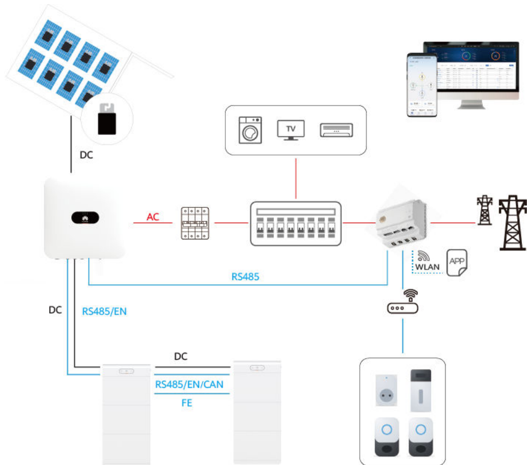
Figura 2-9 Puerto de red conectado al SmartAssistant o al router
