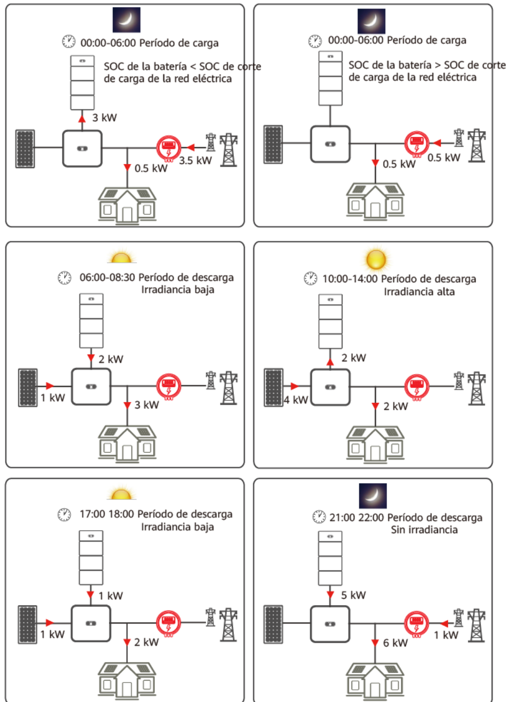
Figura 2-14 Ejemplo de TOU (carga de 00:00 a 06:00 y descarga de 06:00 a 24:00)
