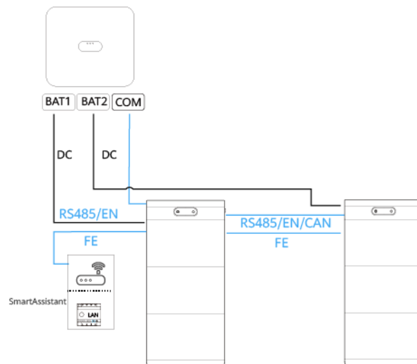
Figura 2-11 Conexión de los ESS al inversor (2)
