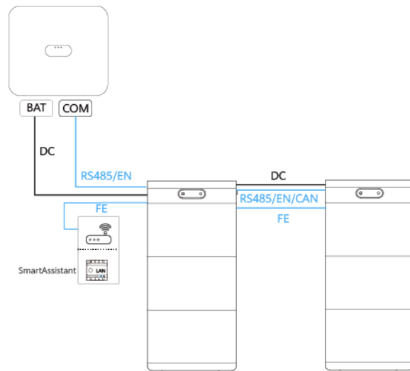
Figura 2-10 Conexión de los ESS al inversor (1)
