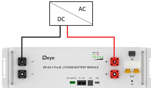
Abbildung 5-2: Einzelbatterieanschluss
